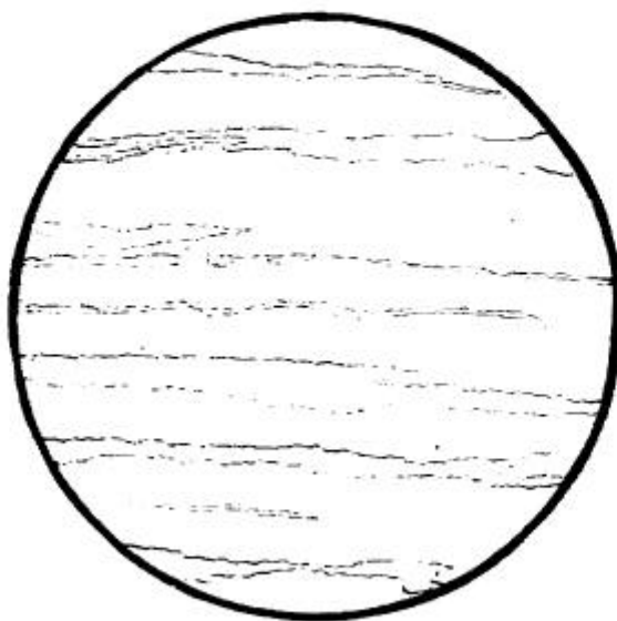
\alpha -相面积 \sim 20\% 3.0 级
