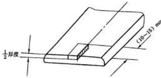
厚度 &gt; 30 mm
