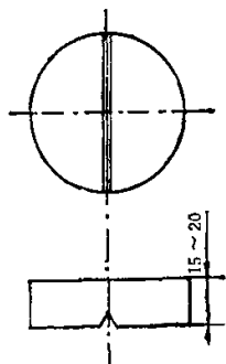
图3 大于40mm条钢纵向断口试样示意图
